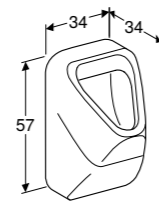
URINOIR Achterinlaat, met keramisch rooster Achterinlaat, met keramisch rooster, KeraTect® Achterinlaat, met keramisch rooster, met vlieg Achterinlaat, met keramisch rooster, met vlieg, KeraTect® Flushcontrol 501 t.b.v. urinoir met achterinlaat
