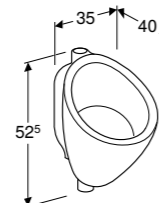
URINOIR 65 Boveninlaat, met keramisch rooster en keramische sifon
