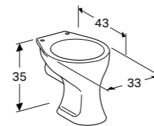
KINDERCLOSET 19 PK Vlakspoel, PK
