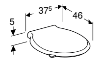
CLOSETZITTING Doorlopend scharnier Standaard bevestiging
