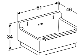
GOOTSTEEN 61 CM
