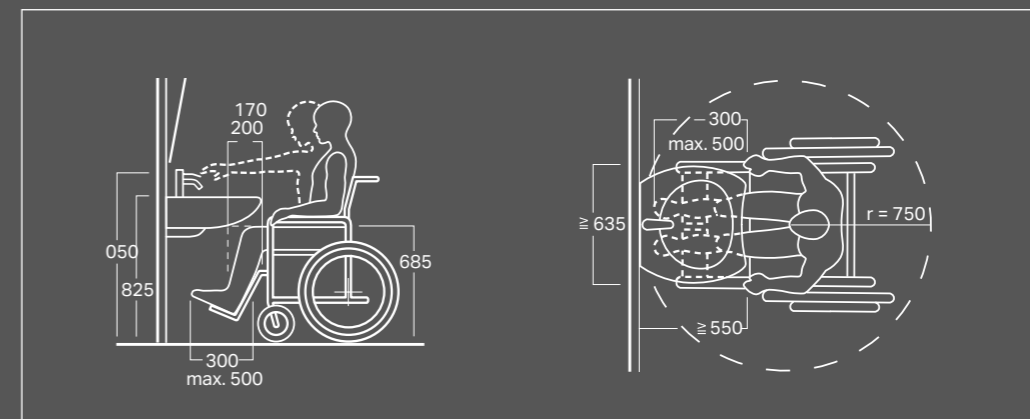
Voorbeeld wastafelopstelling voor rolstoelgebruikers
