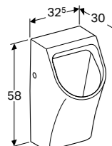
URINOIR 90 Achterinlaat Flushcontrol 1000 t.b.v. urinoir 90/92
