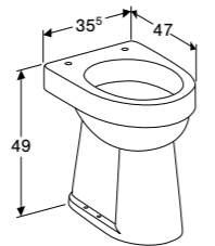
STAAND CLOSET 84 Vlakspoel, AO, verhoogd 49 cm Vlakspoel, PK, verhoogd 49 cm
