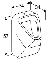
URINOIR Boveninlaat Boveninlaat, KeraTect® Boveninlaat, met vlieg Boveninlaat, met vlieg, KeraTect®
