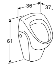
URINOIR 40 Achterinlaat Boveninlaat Flushcontrol 501 t.b.v. urinoir met achterinlaat
