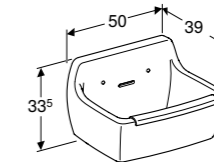
NORMA GOOTSTEEN
