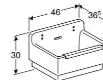
GOOTSTEEN 46 CM
