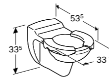
KINDERWANDCLOSET Diepspoel met 2-delige dijstukken, rood
